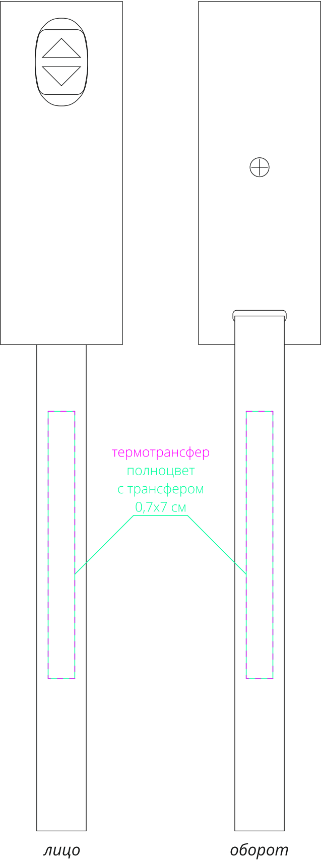
ручка M1:1
